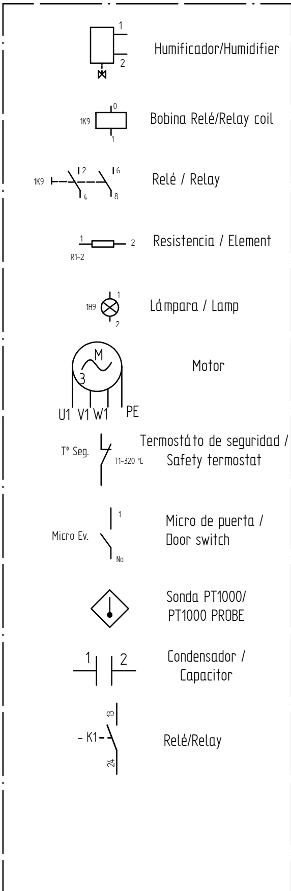
Esquema eléctrico/Electric scheme modelo/model RG 311
