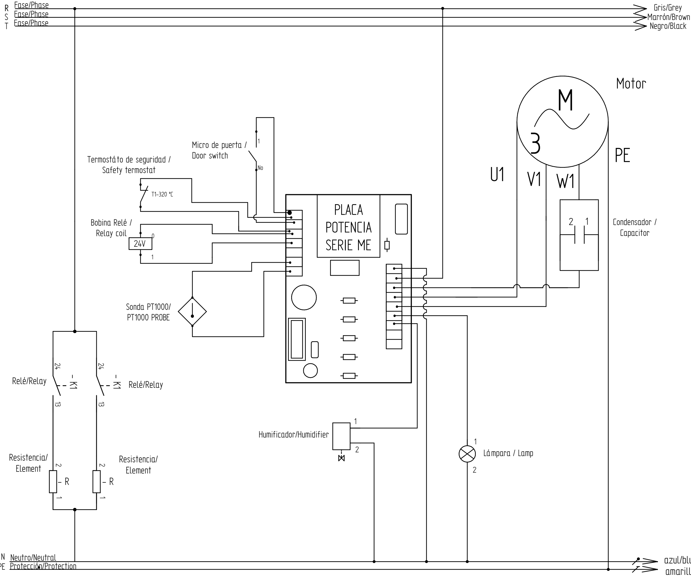
Esquema eléctrico/Electric scheme modelo/model RG 611
