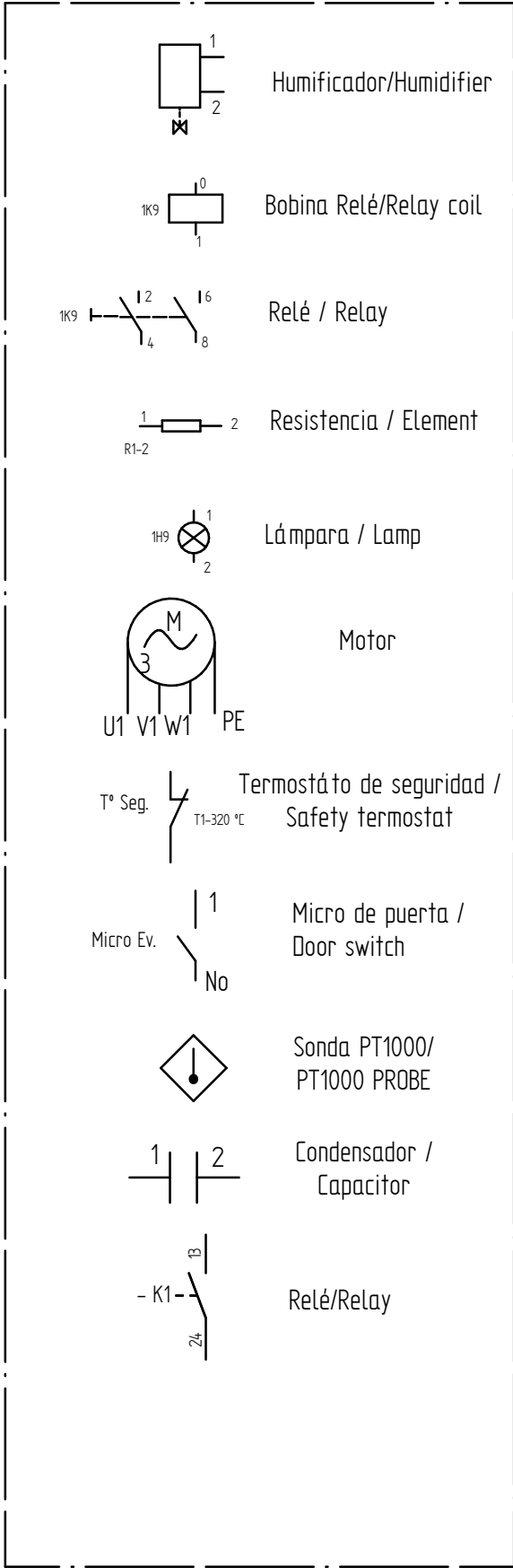
Esquema eléctrico/Electric scheme modelo/model RG 611
