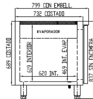
SECCIÓN SIN ENCIMERA
