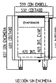
SECCIÓN SIN ENCIMERA
