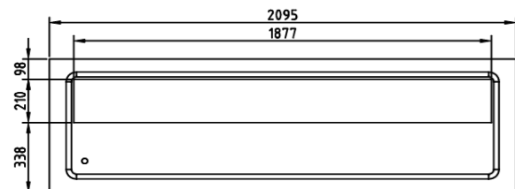
VUE INFÉRIEURE
