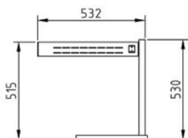
ÉLEVATION
