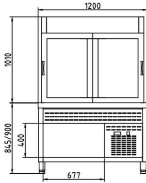
ÉLÉVATION
