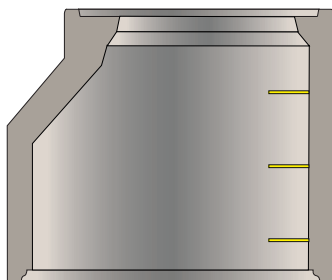
Cône réducteur H 90cm avec ou sans échelon
