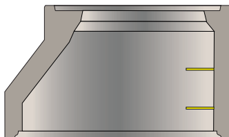
Cône réducteur H 60cm avec ou sans échelon
