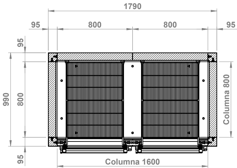
SECCIÓN E-E ESCALA 1 : 25
