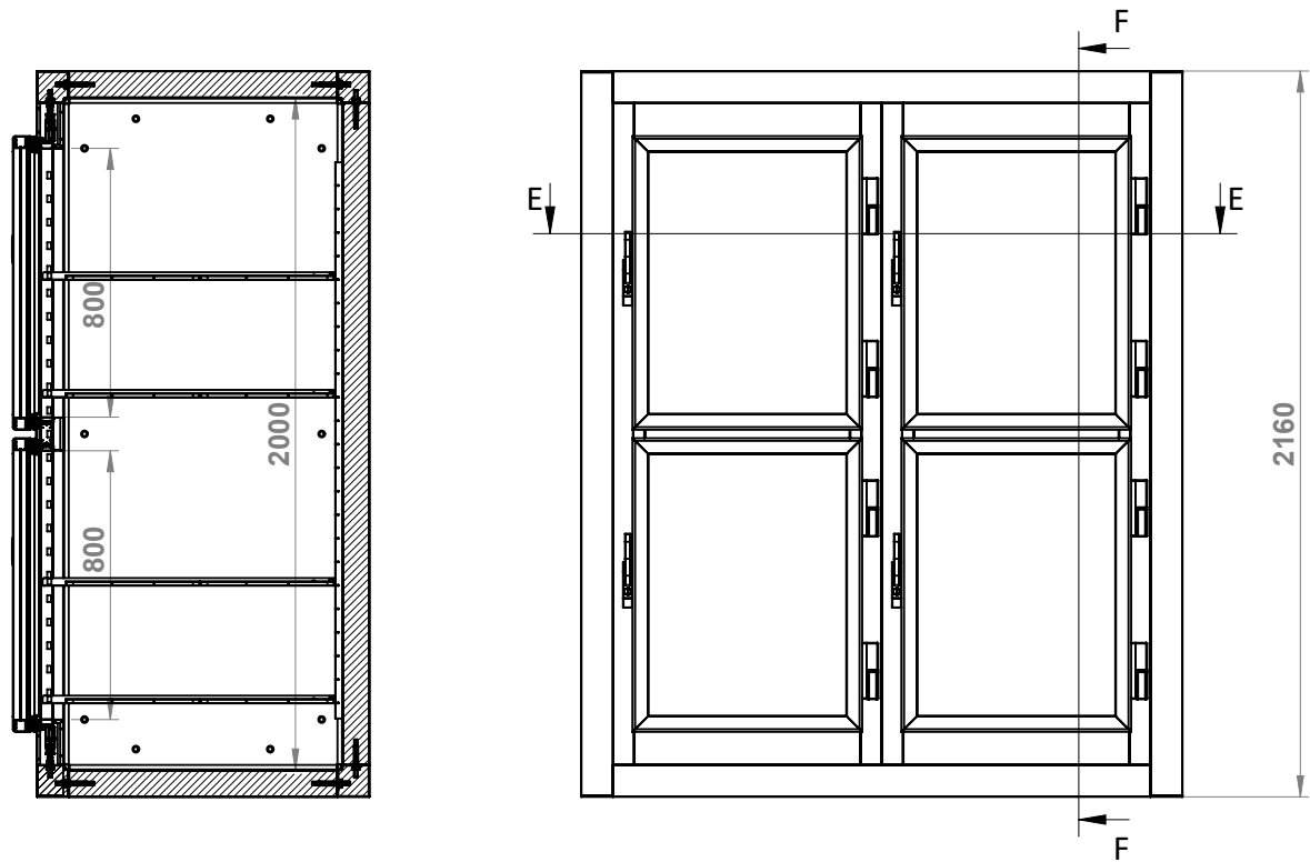
SECCIÓN F-F ESCALA 1 : 25
