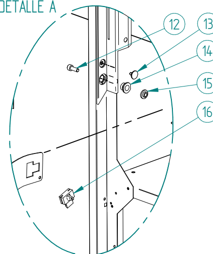
DETALLE A
