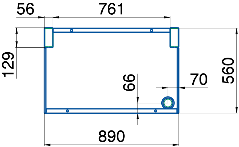
Panel cutout for stopper / Overlapping Hueco de montaje de tampón / acaballado
