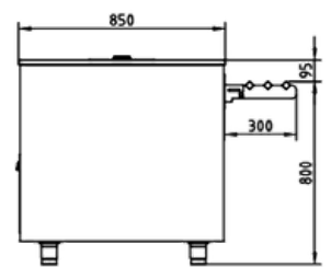
PROFILÉ
