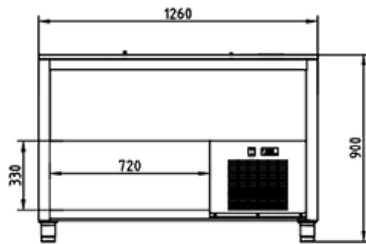
ÉLÉVATION
