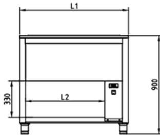
ÉLÉVATION
