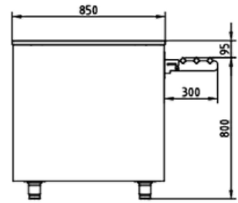
PROFILÉ
