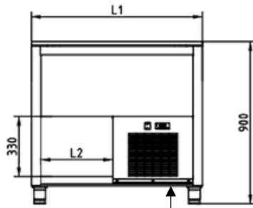
ÉLÉVATION
