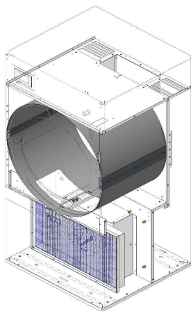
IMPIANTO ASPIRAZIONE SUCTION SYSTEM
