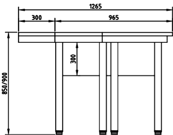
ÉLÉVATION
