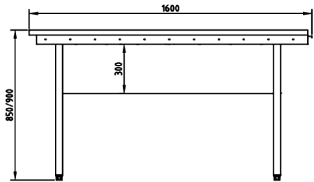
ÉLEVATION
