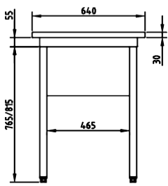
PROFILÉ
