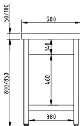
ÉLÉVATION
