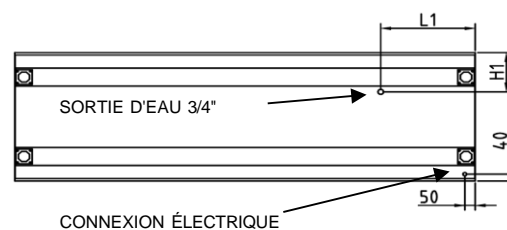
VUE INFÉRIEURE
