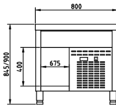
ÉLÉVATION
