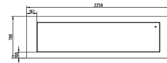
VUE INFÉRIEURE
