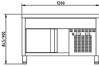
ÉLÉVATION
