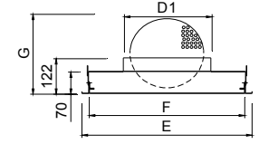
Plénum avec piquage supérieur
